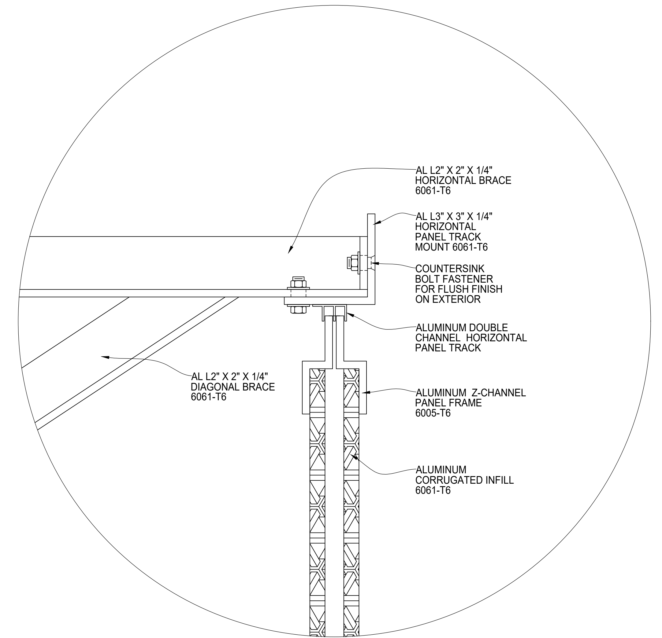
DETAIL ~ A-A
