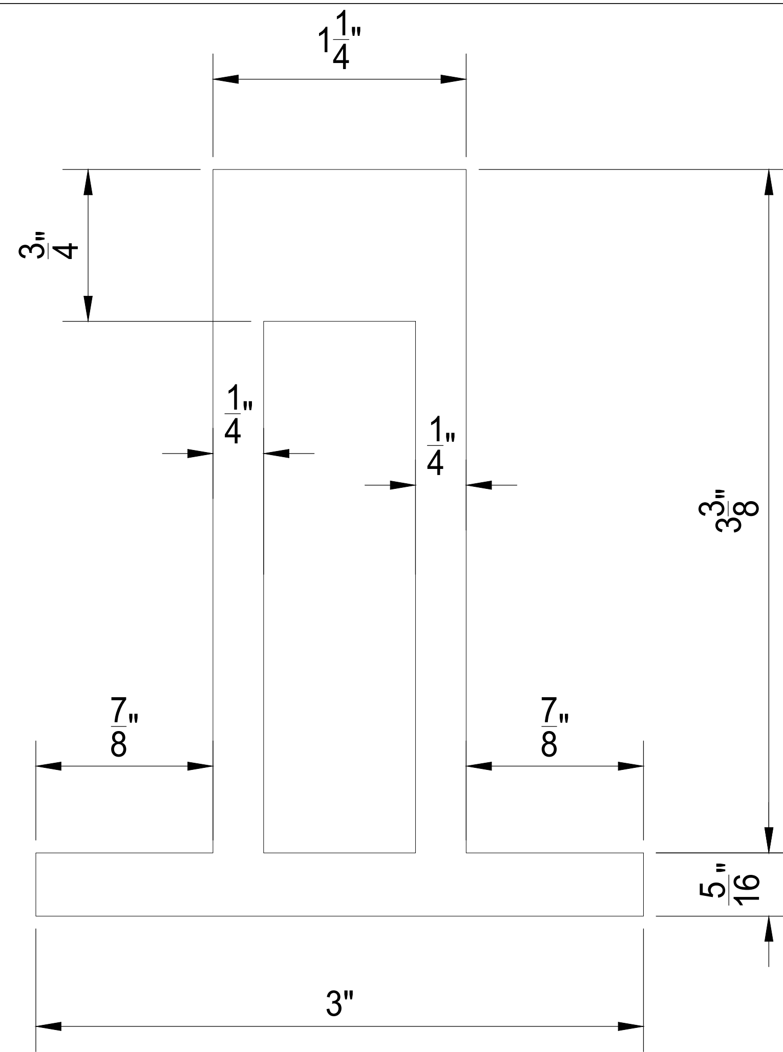
TUBULAR T-POST
